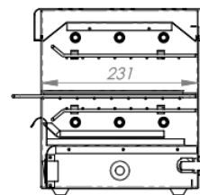
SECCIÓN A-A
