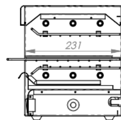
SECCIÓN A-A
