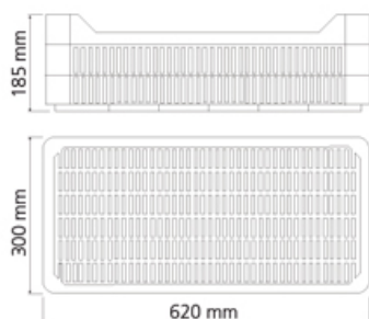
Cesta Inferior (CIA600)
