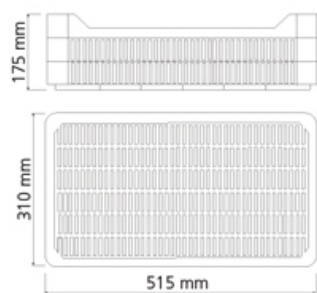
Cesta Superior (CSA600)
